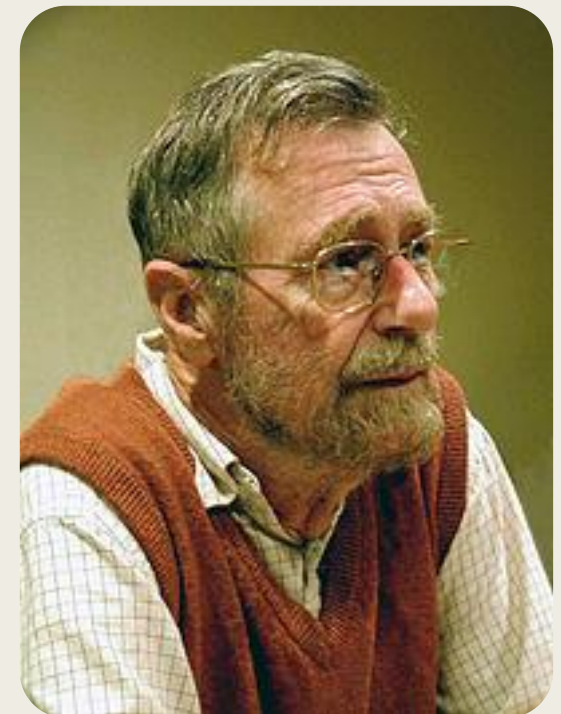
Edsger Dajkstra
